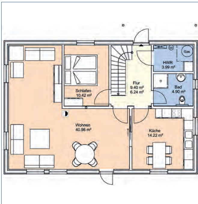
Erdgeschoss
