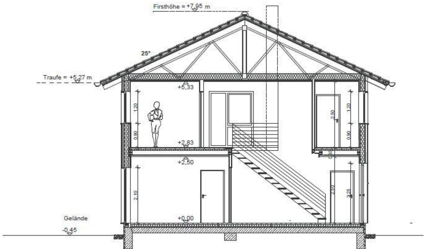
Querschnitt (Standart) - Darstellung mit 2 Vollgeschossen
